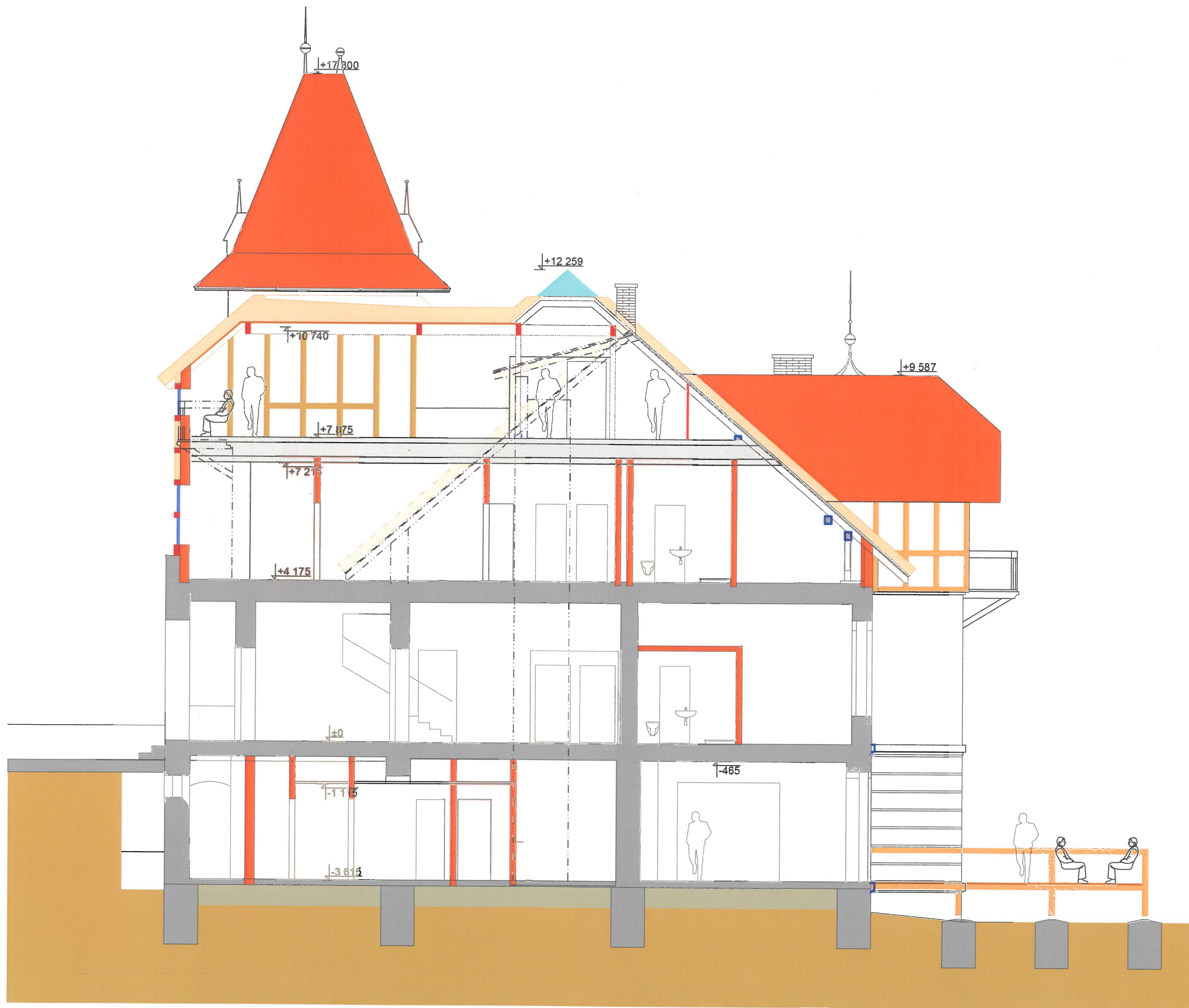
LOMENÝ ŘEZ VE SMĚRU SEVER - JIH
